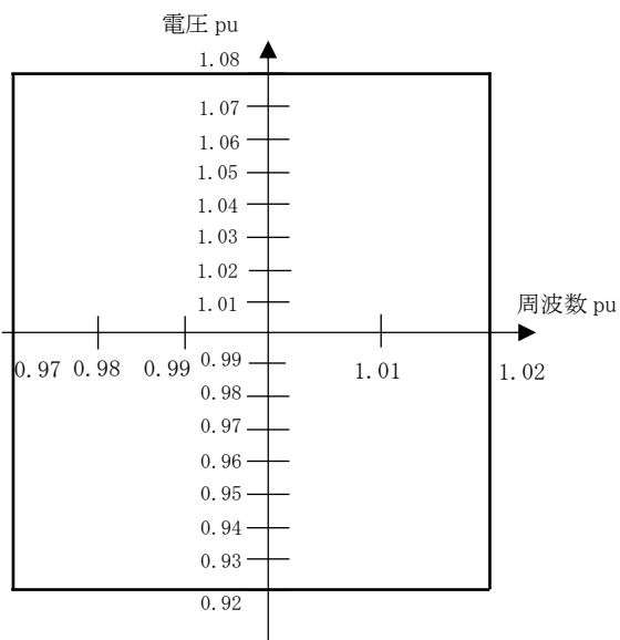
逆変換装置
